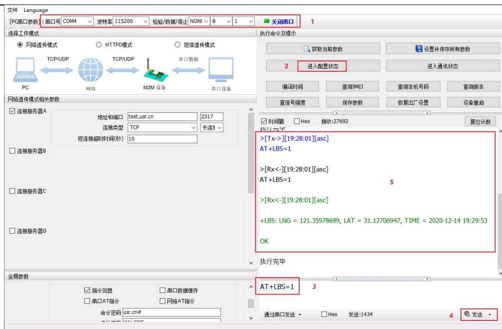
图 20. 查询基站信息
