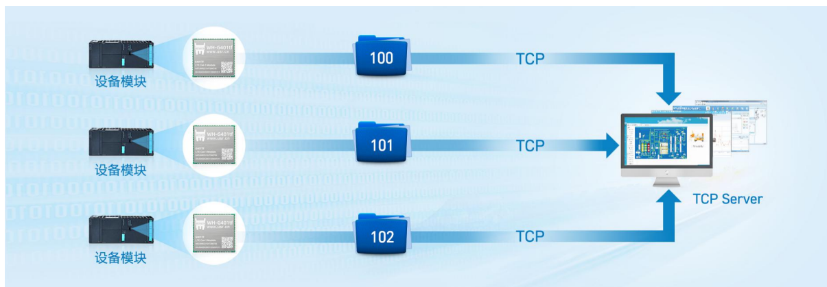
图 10. 注册包功能示意图
