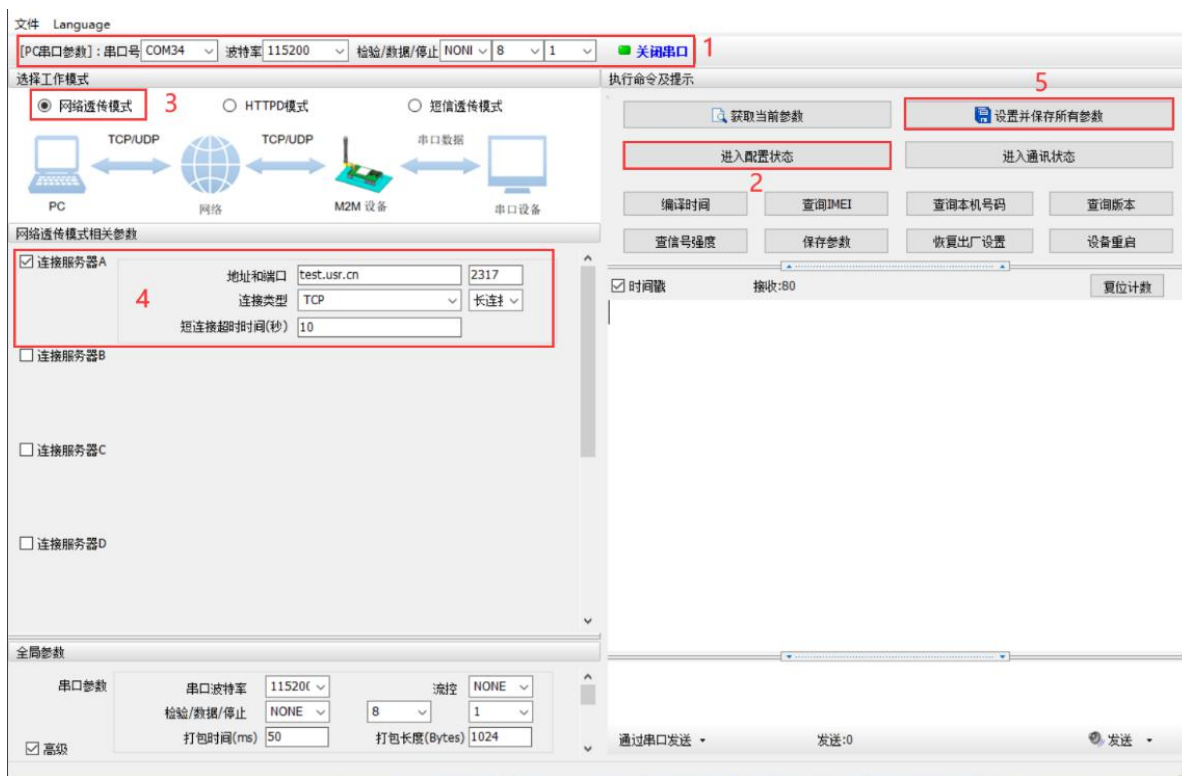
图 5. 设置软件示意图
